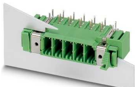
С разворотом на 180°, резьбовой фланец, проходная деталь для подключения экрана на внутренней стороне устройства
