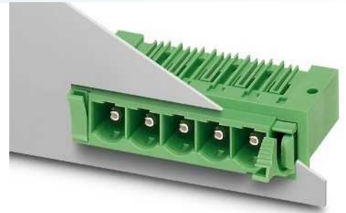
Без резьбового фланца
